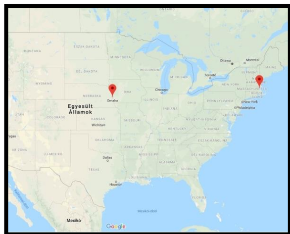
19. ábra: Milgram kísérleteinek kiinduló- és célállomásai forrás: Google Earth
