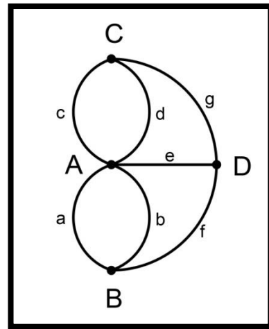
18. ábra: A königsbergi hidak gráfokká alakított alapesete [60]
