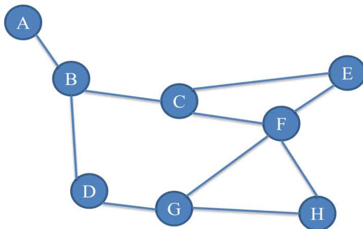
23. ábra: Példagráf (saját szerkesztés)
