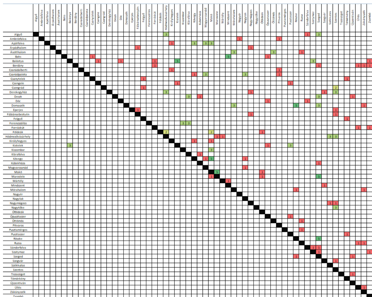
44. ábra: Csongrád megye településstruktúrájának kapcsolati mátrixa (saját szerkesztés)
